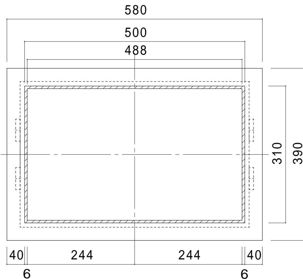
背面図( 扉 B )
