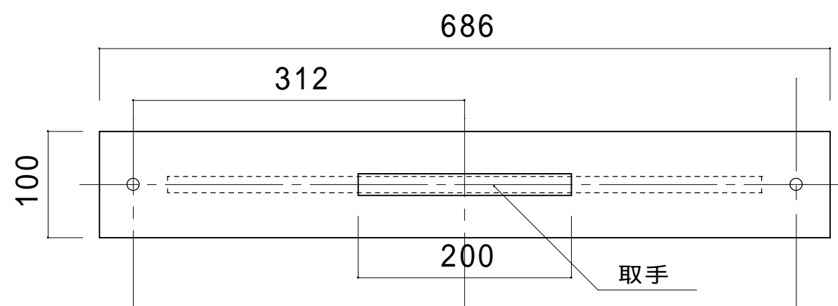
正面図( 鉄板出入口蓋 )
