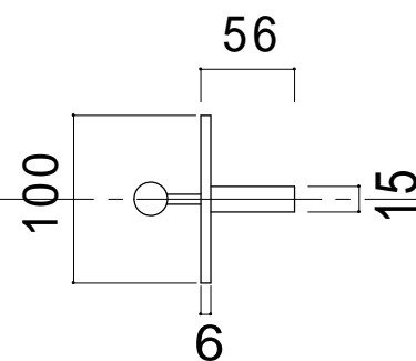
側面図( 鉄板出入口蓋 )
