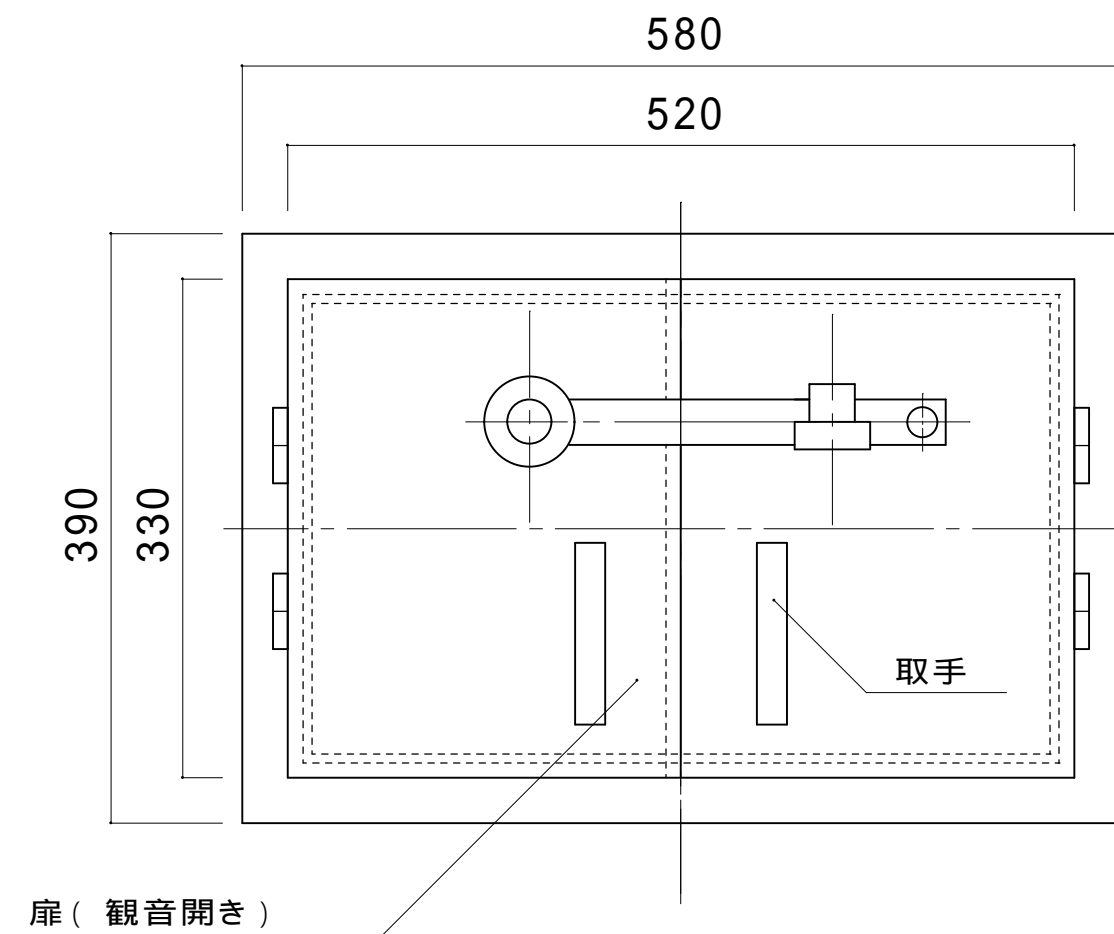
正面図( 扉 B )
