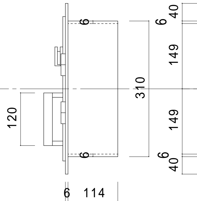
側面図( 扉 B )
