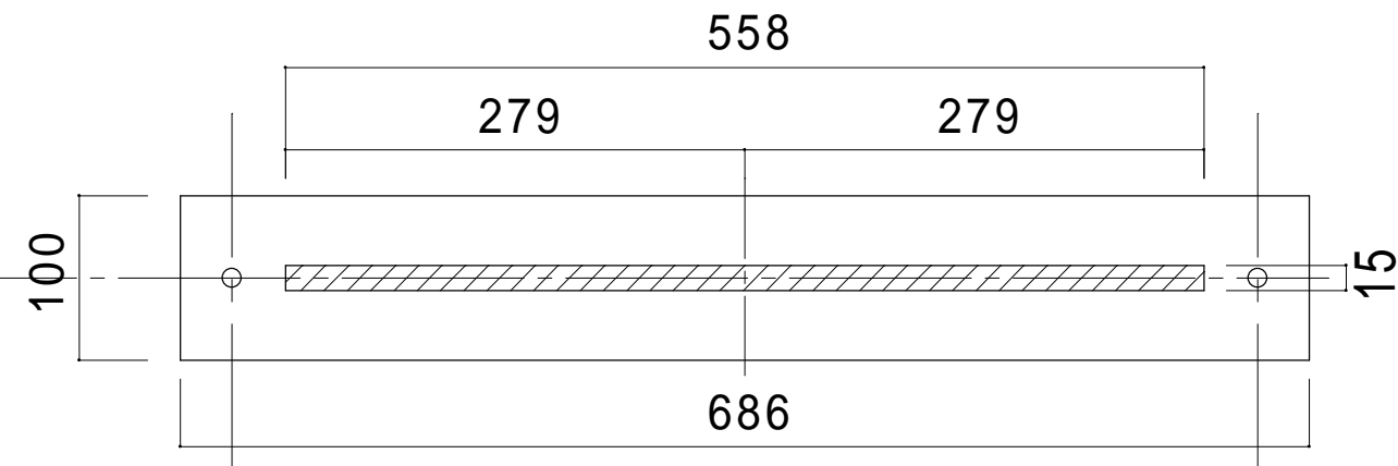
背面図( 鉄板出入口蓋 )
