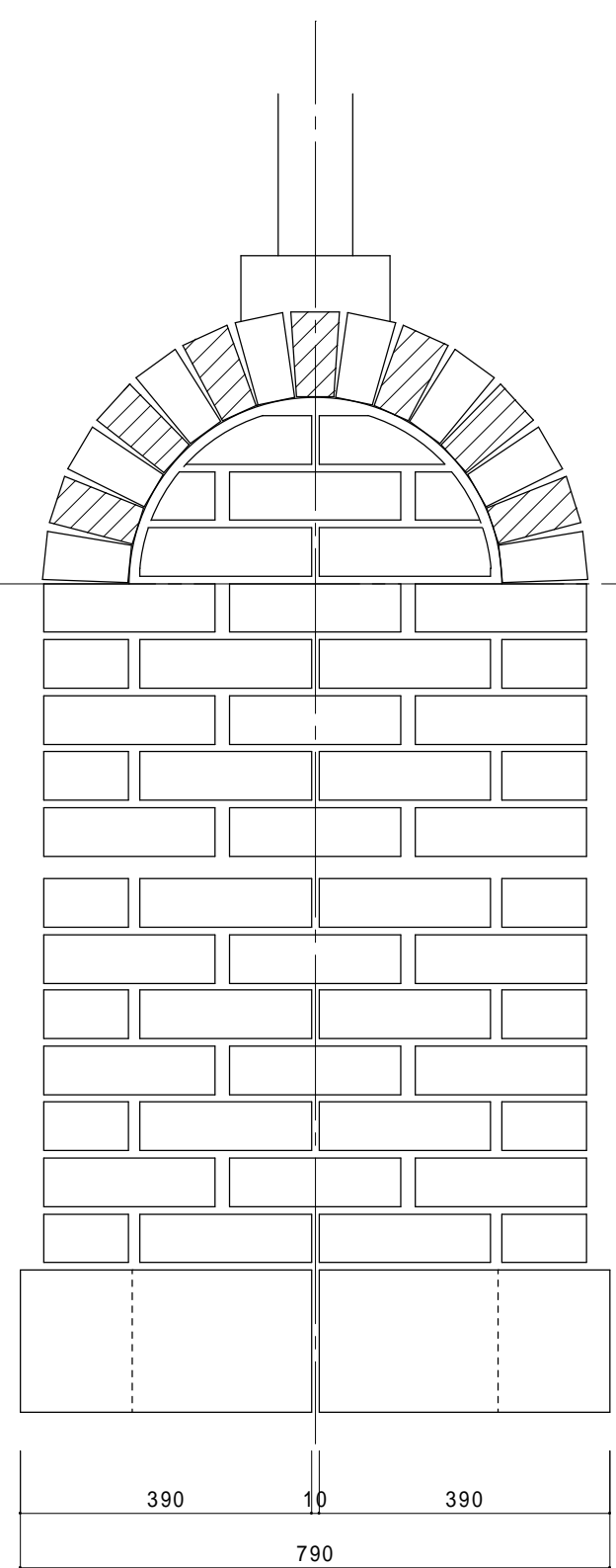
背面図
