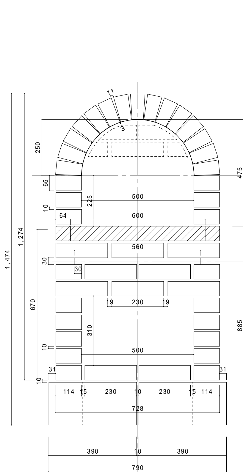
正面図
