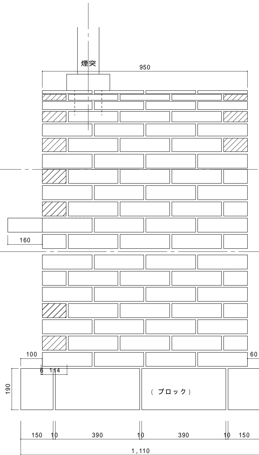
右側面図
